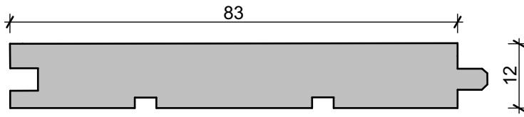
TNZ T & G
